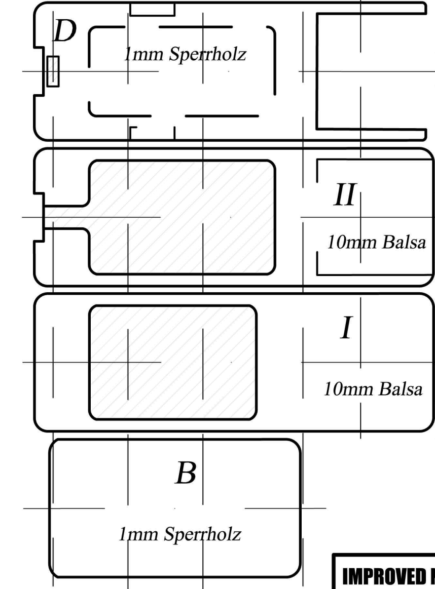
Bugmodul
