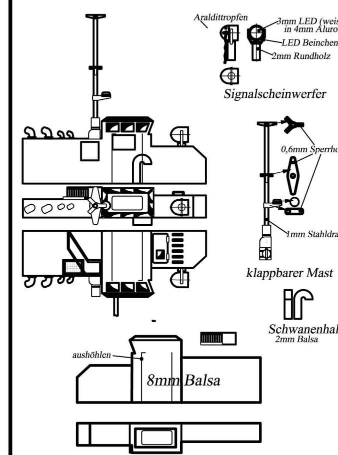
Deckshaus
