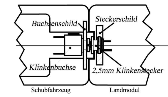
Klinkensteckerkupplung zwischen Einheiten
